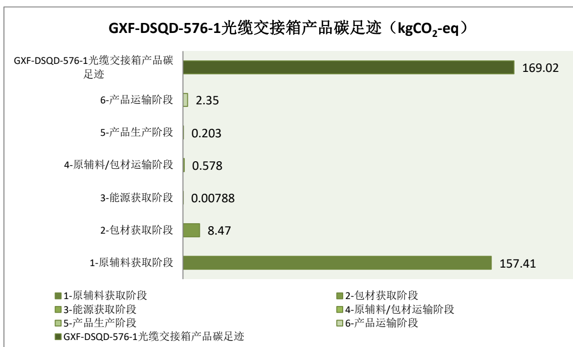
图 10 GXF-DSQD-576-1 光缆交接箱产品生命周期总图
