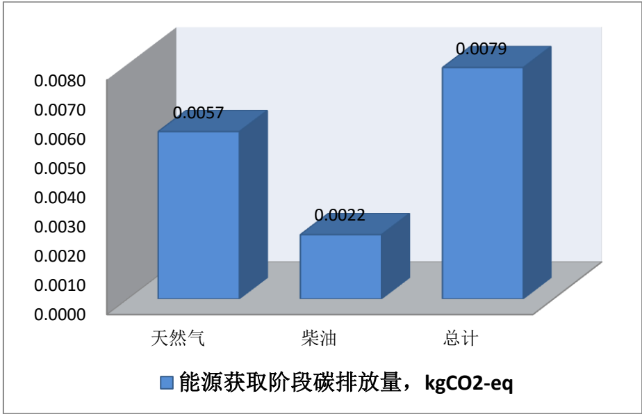
图 5 能源获取阶段
