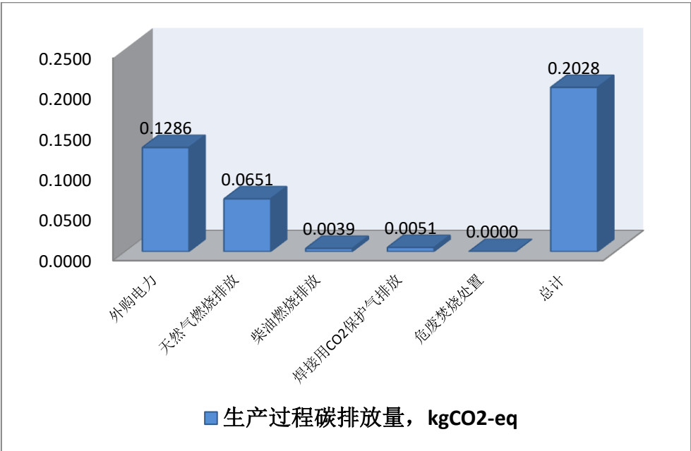
图 7 产品生产阶段
