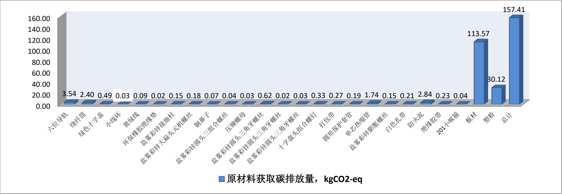
图 3 原辅料获取阶段
