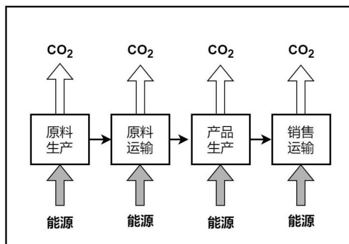
图 2 GXF-DSQD-576-1 光缆交接箱产品生命周期评价边界图
