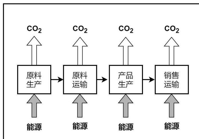
图 2 HRT-ZHJZJ-01 综合集装架产品生命周期评价边界图
