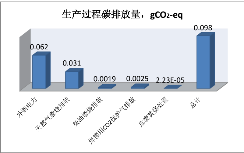
图 6 产品生产阶段
