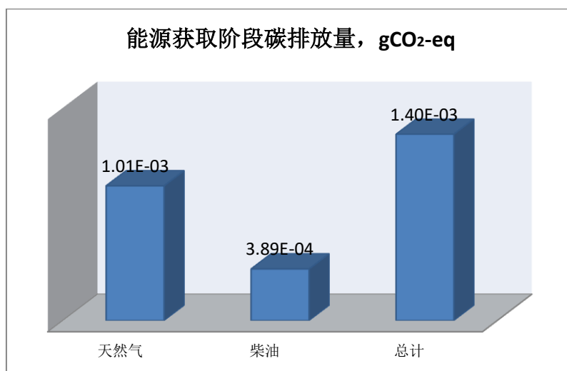
图 4 能源获取阶段
