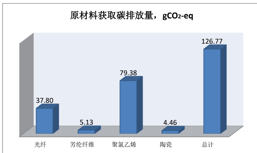
图 3 原辅料获取阶段
