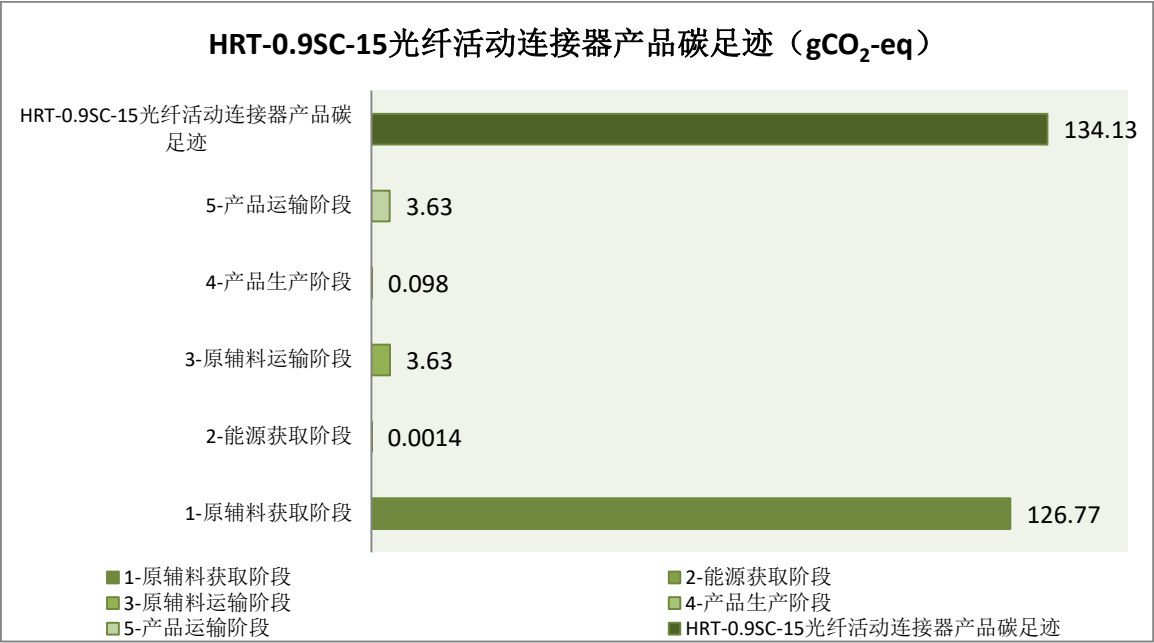
图 9 HRT-0.9SC-15 光纤活动连接器产品生命周期总图
