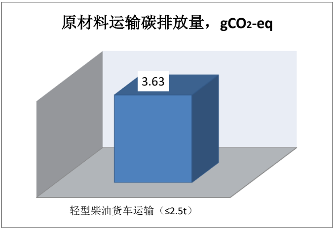
图 5 原辅料运输阶段
