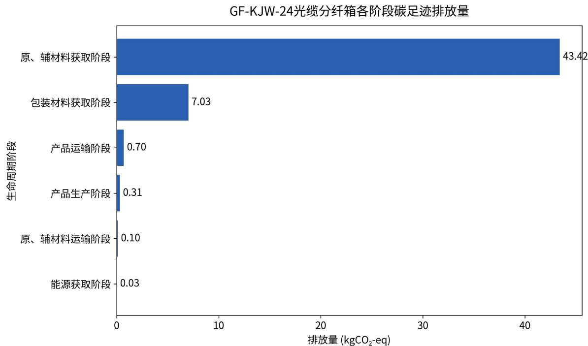
图 4 GF-KJW-24 光缆分纤箱产品生命周期总图
