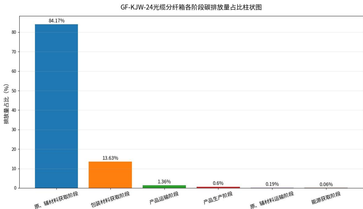
图 5 各阶段碳排放量占比图
