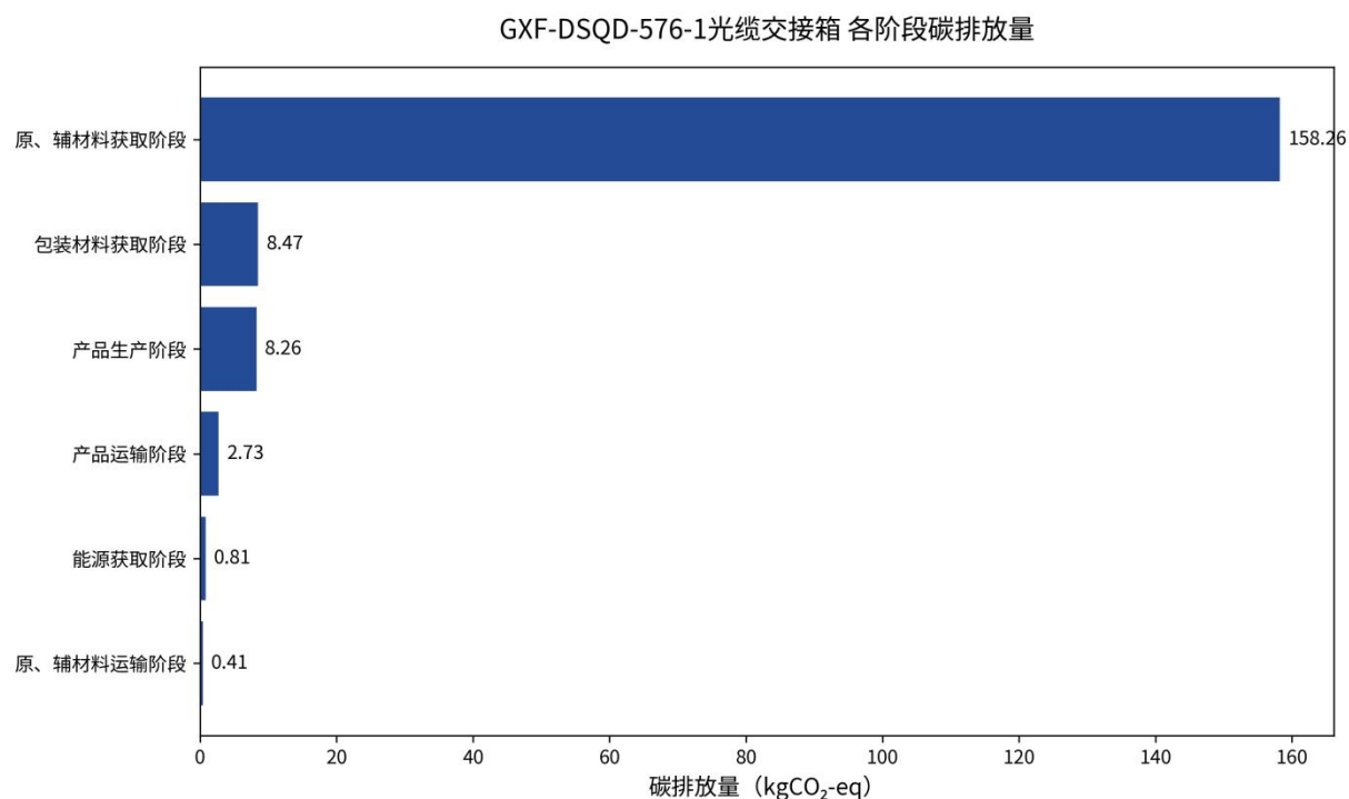
图 4 GXF-DSQD-576-1 光缆交接箱产品生命周期总图
